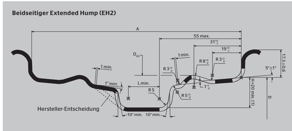
Diese Kontur ist gültig für Felgengrößen von 5 ½ J bis 13 ½ J (1): H \geq 22 notwendig für automatische Montage - beide Wulste gleichzeitig
